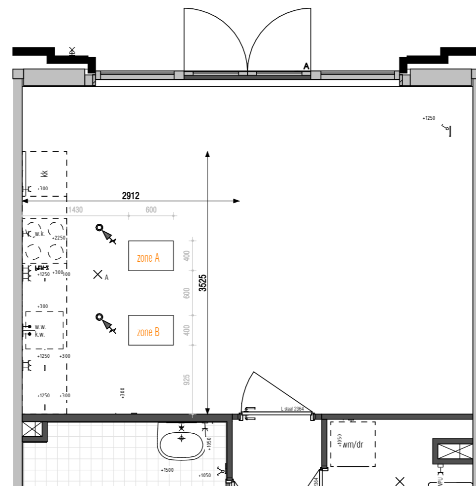
476302 keukenpositie 2
