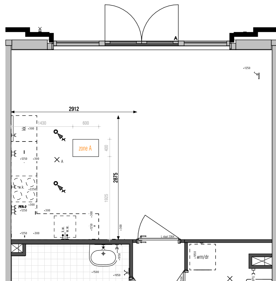
476304 keukenpositie 4 (standaard type B1)
