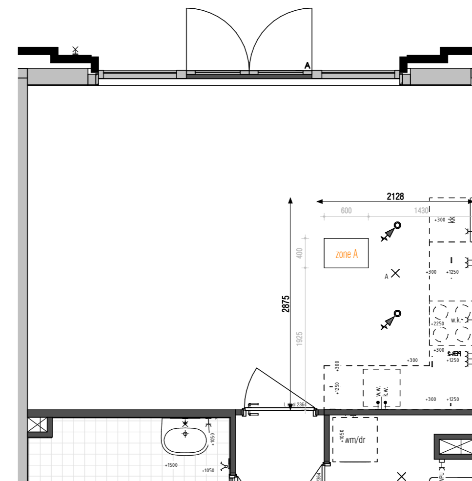
476303 keukenpositie 3 (standaard type B2)
